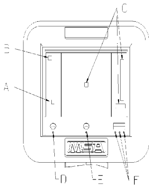
Figure 4. Interface utilisateur de l'Evolution 5200 et l'Evolution 5200HD²
